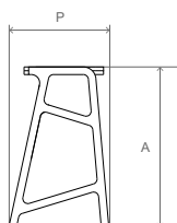
Vista Lateral
